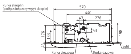
WIDOK A
